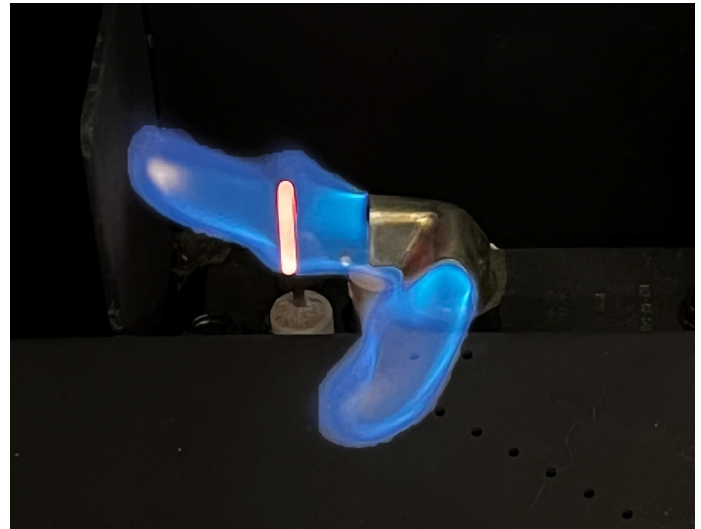
Figure 2: Flamme du pilote Proflame II
