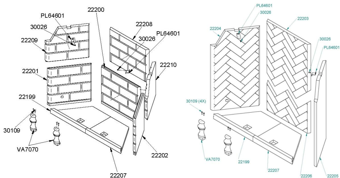
Figure 38 – Vues explosés des panneaux réfractaires du foyer FP11 Frontenac
