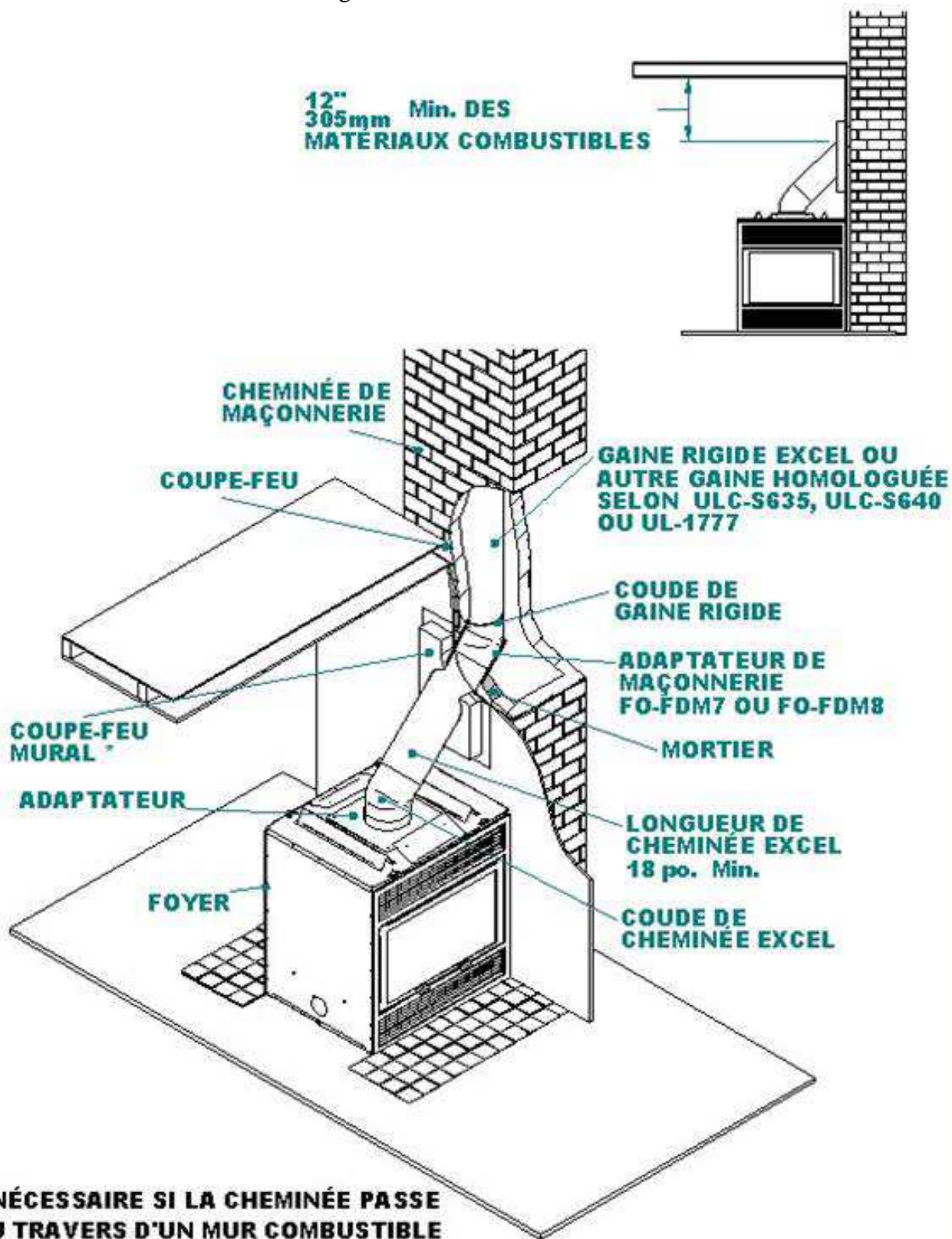
Figure 5 : Cheminée EXCEL
